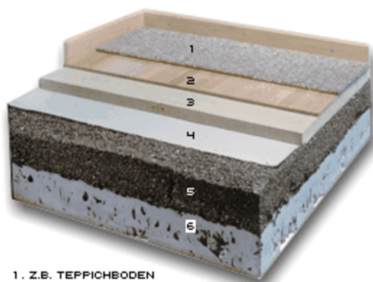
1. Z.B. TEPPICHBODEN 2. PARKETT/LAMINAT 3. BODENVERLEGEPLATTE MIN. 22mm 4. WELLPAPPE 5. VERMIBIT TROCKENAUSGLEICHSCÜTTUNG 6. ROHBETONDECKE
